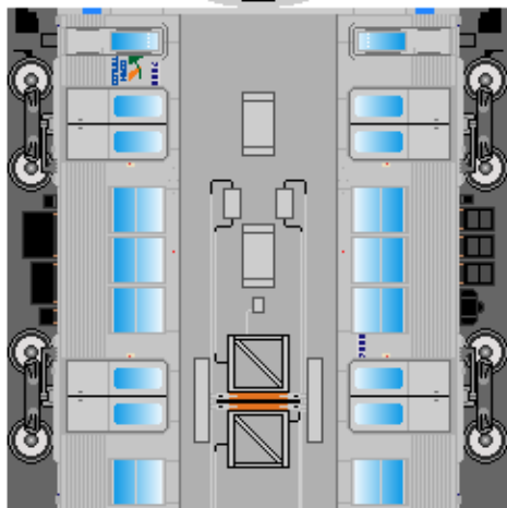
③ デハ7023 (弘南線)
